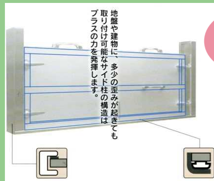
サイド柱 ステンレス魔法瓶のような二重構造のサイド柱により、地盤や建物に多少の歪みが起きていても取り付け可能な上、ロックによる圧着にも柔軟性を発揮しています。
