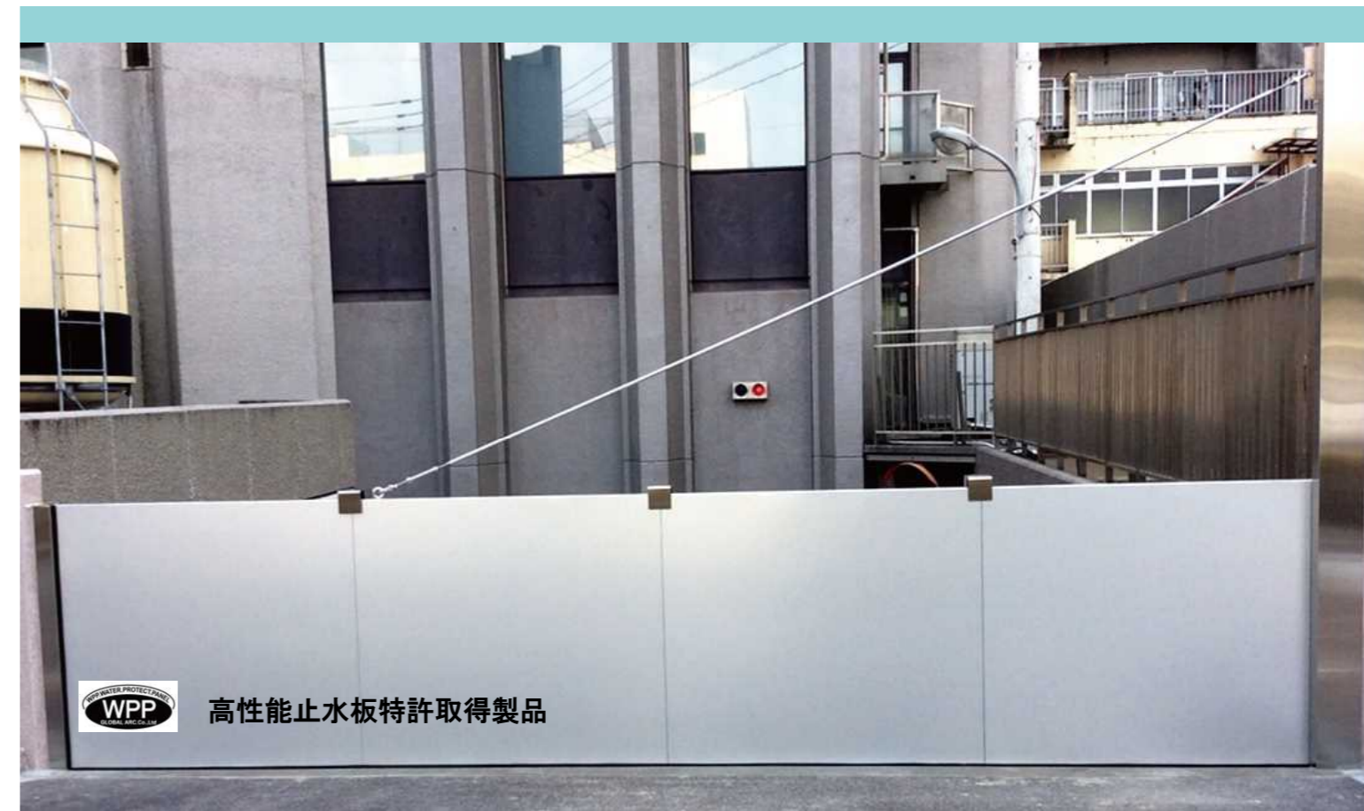
宮崎銀行 本店 スイング式 w 5,420×H 1,200
